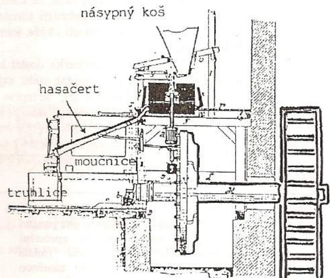
Schéma vodního mlýna o jednom mlýnském „složení“
